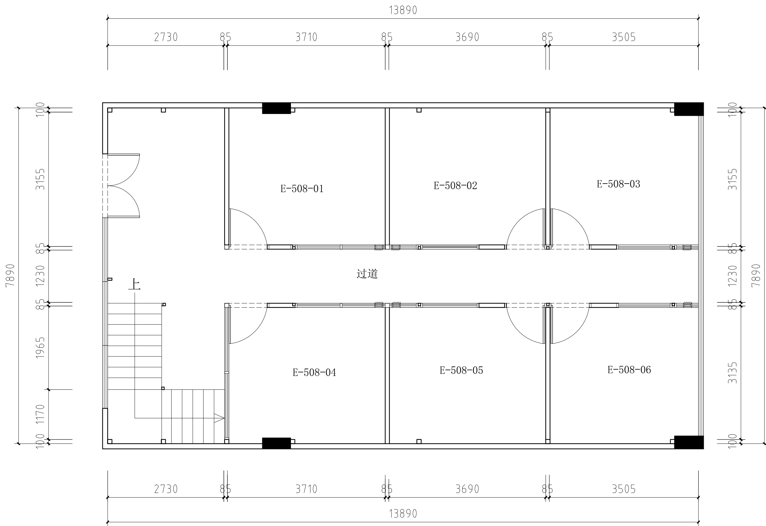
E508一层平面图
