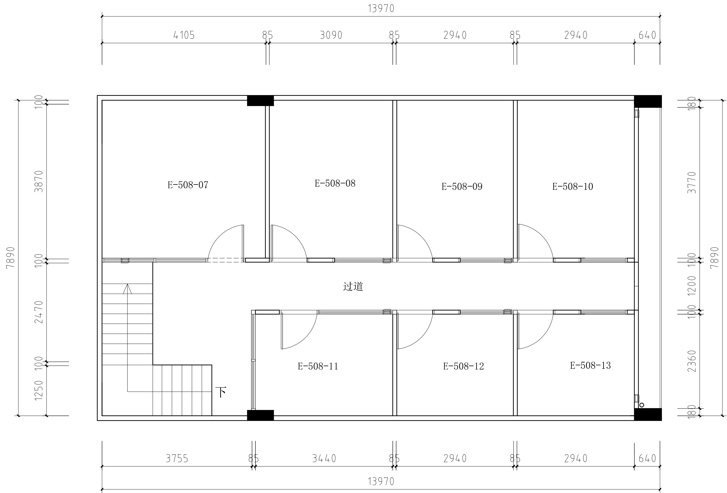
E508夹层平面图
